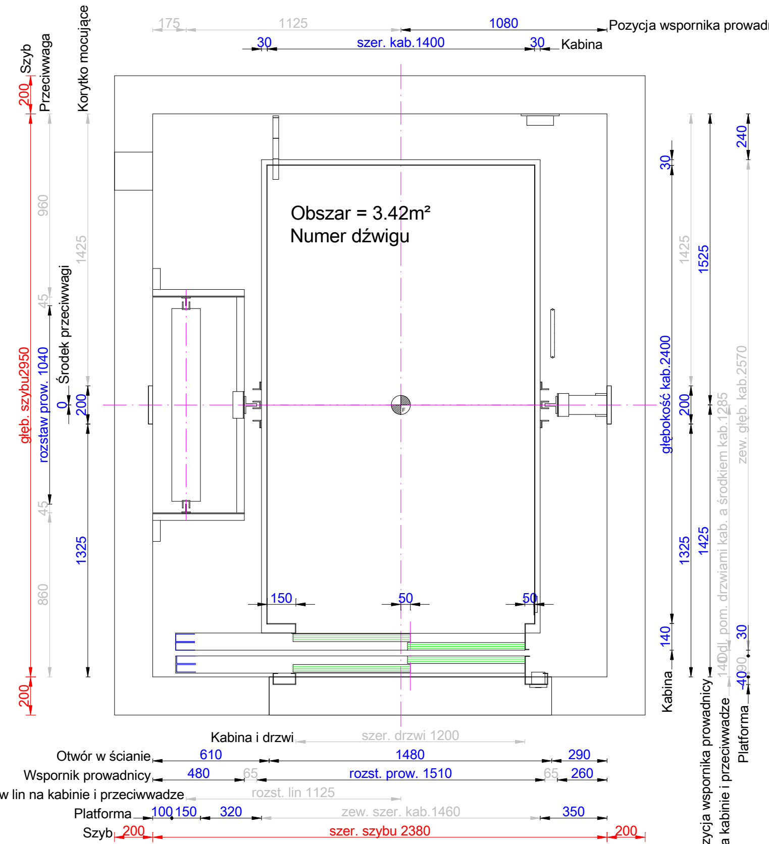
Schemat szybu Skala: 1:20
